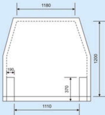
PORTALE POSTERIORE CON PORTE SUPPLEMENTARI (OPTIONAL) REAR DOOR FRAME WITH SUPPLEMENTARY DOORS (OPTIONAL) PORTAIL POSTÉRIEUR AVEC PORTES SUPPLÉMENTAIRES (OPTIONAL) PORTON TRASERO CON PUERTAS SUPLEMENTARIAS (OPCIONAL)
