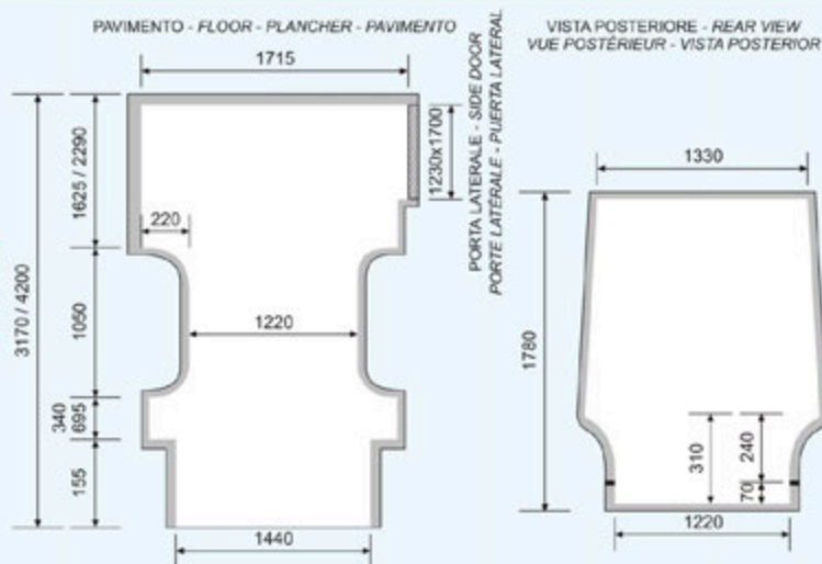
PORTALE POSTERIORE CON PORTE SUPPLEMENTARI (OPTIONAL) REAR DOOR FRAME WITH SUPPLEMENTARY DOORS (OPTIONAL) PORTAL POSTÉRIEUR AVEC PORTES SUPPLÉMENTAIRES (OPTIONAL) PÓRTON TRASERO CON PUERTAS SUPLEMENTARIAS (OPCIONAL)
