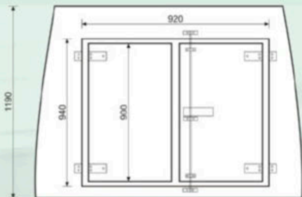
PORTALE POSTERIORE CON PORTE SUPPLEMENTARI (OPTIONAL) REAR DOOR FRAME WITH SUPPLEMENTARY DOORS (OPTIONAL) PORTAIL POSTÉRIEUR AVEC PORTES SUPPLÉMENTAIRES (OPTIONAL) PORTON TRASERO CON PUERTAS SUPLEMENTARIAS (OPCIONAL)
