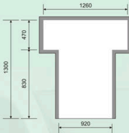
PAVIMENTO - FLOOR - PLANCHER - PAVIMENTO
