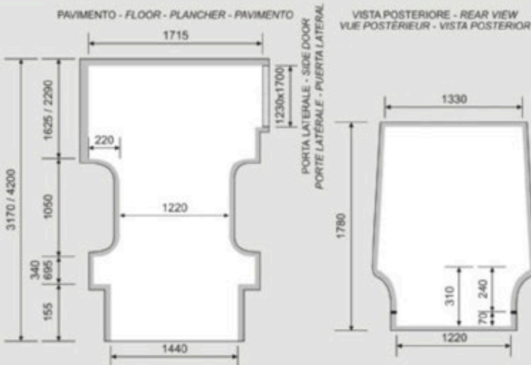
PORTALE POSTERIORE CON PORTE SUPPLEMENTARI (OPTIONAL) REAR DOOR FRAME WITH SUPPLEMENTARY DOORS (OPTIONAL) PORTAL POSTÉRIEUR AVEC PORTES SUPPLÉMENTAIRES (OPTIONAL) PORTON TRASERO CON PUERTAS SUPLEMENTARIAS (OPCIONAL)
