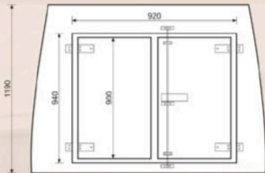
PORTALE POSTERIORE CON PORTE SUPPLEMENTARI (OPTIONAL) REAR DOOR FRAME WITH SUPPLEMENTARY DOORS (OPTIONAL) PORTAL POSTÉRIEUR AVEC PORTES SUPPLÉMENTAIRES (OPTIONAL) PORTON TRASERO CON PUERTAS SUPLEMENTARIAS (OPCIONAL)
