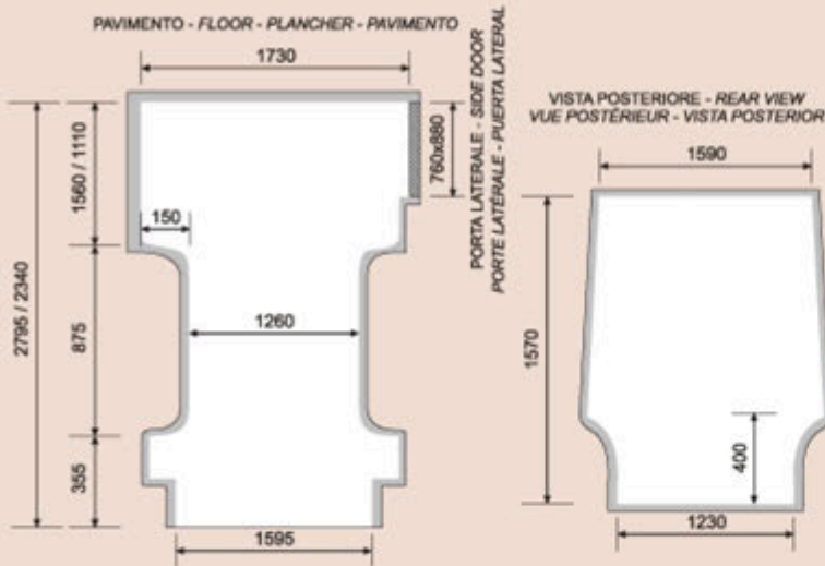
PORTALE POSTERIORE CON PORTE SUPPLEMENTARI (OPTIONAL) REAR DOOR FRAME WITH SUPPLEMENTARY DOORS (OPTIONAL) PORTAIL POSTÉRIEUR AVEC PORTES SUPPLÉMENTAIRES (OPTIONAL) PUERTA TRASERO CON PUERTAS SUPLEMENTARIAS (OPCIONAL)
